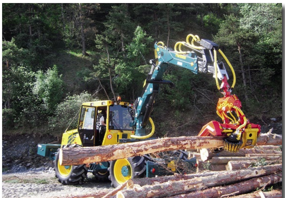
HSM 904 im Einsatz: Der Harvesteraufbau, vorne am Greifarm, entfernt die Äste eines Baumstamms.
